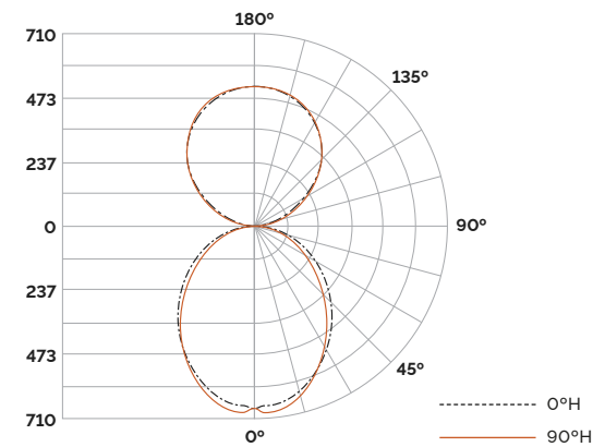
TALLDI-4-400-375-SD-CL-35K (80+ CRI)
