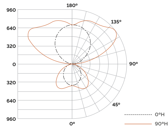
TALLDI-4-325-750-WD-BW-35K (80+ CRI)
