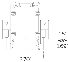
9/16" T-Bar Flush
