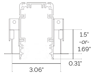
15/16" T-Bar Tegrular
