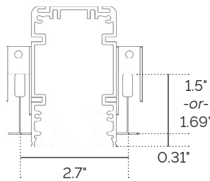
9/16" T-Bar Tegrular
