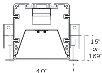
9/16" T-Bar Flush
