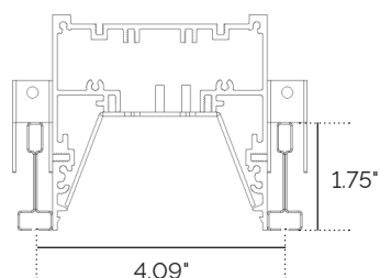
9/16" T-Bar Tegular
