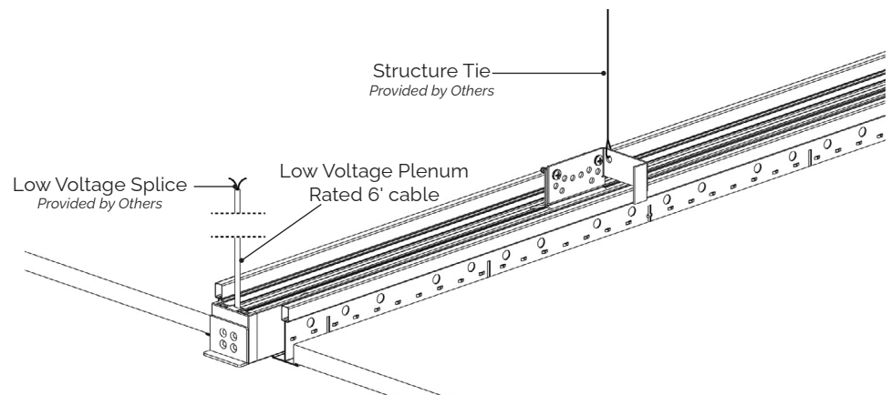
9/16" T-Bar
