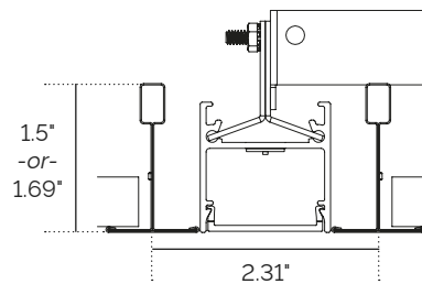
15/16" T-Bar
