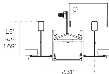
9/16" T-Bar
