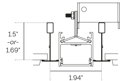
9/16" T-Bar
