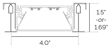
9/16" T-Bar Flush
