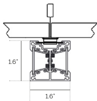
TB1 9/16" T-Bar
