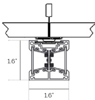
TB2 15/16" T-Bar
