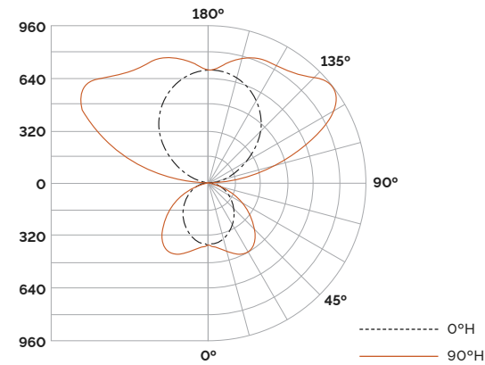
TALLDI-4-325-750-WD-BW-35K (80+ CRI)
