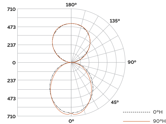
TALLDI-4-400-375-SD-CL-35K (80+ CRI)
